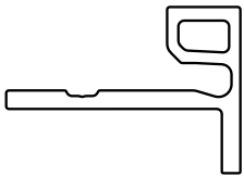
Bordure de finition UH50 75 x 54 mm (3.0 x 2.1 po)
