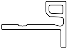
Bordure de finition UH50 75 x 54 mm (3.0 x 2.1 po)
