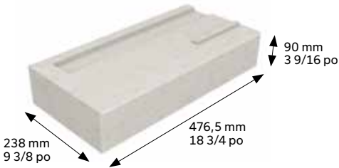
MODULE DE COIN LONG - GAUCHE
