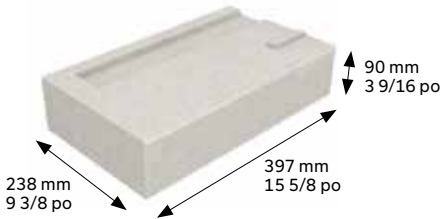
MODULE DE COIN MOYEN - GAUCHE
