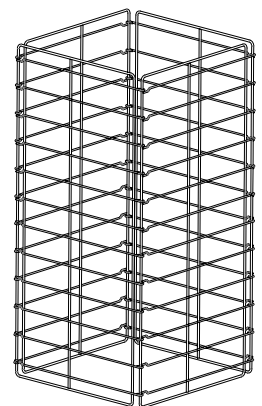
GRILLE TANDEM POUR COLONNE
