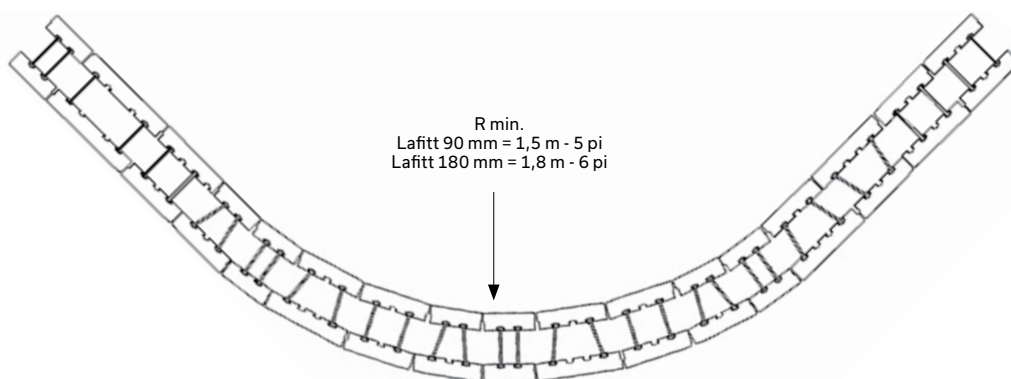
MURET AVEC CONNECTEUR DE PLASTIQUE
