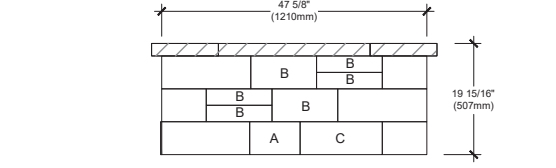
ELEVATION A
