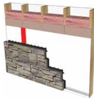
Charpente standard avec OSB ou contre-plaqué
